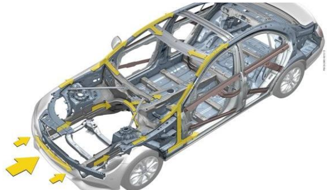
Transmisión de fuerzas durante una colisión
